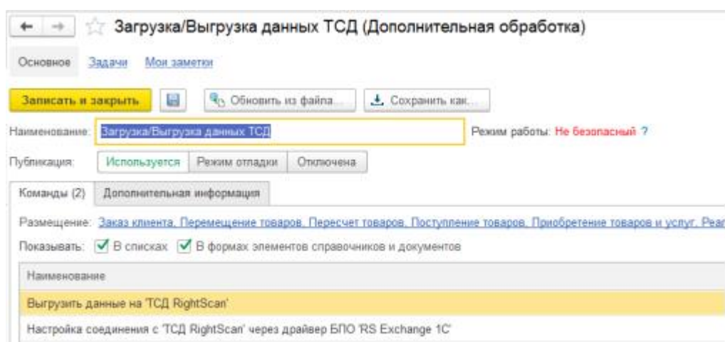
Рис. 1.19 Окно настройки внешней обработки
